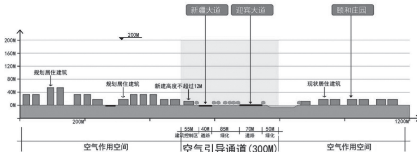
图5 迎宾大道一级通风廊道剖面图
