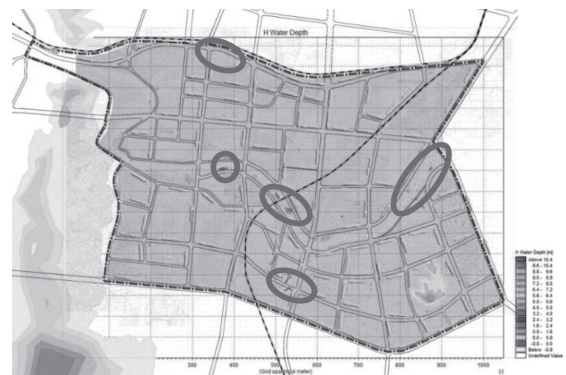
图7 GIS软件模拟降雨后积水程度分布图
